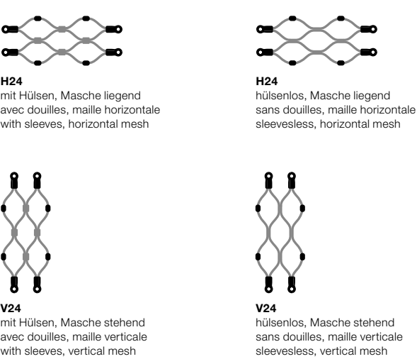
Reguläre Randausbildungen am Webnet Finitions de bords standards sur Webnet Regular perimeter types for Webnet
