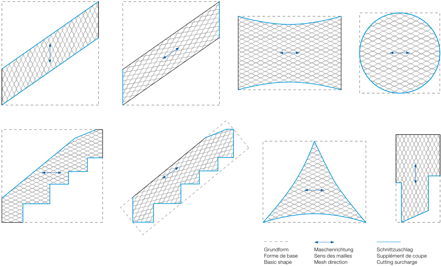
Beispiele für Webnet-Sonderformen Exemples de formes spéciales de Webnet Examples of Webnet special shapes
